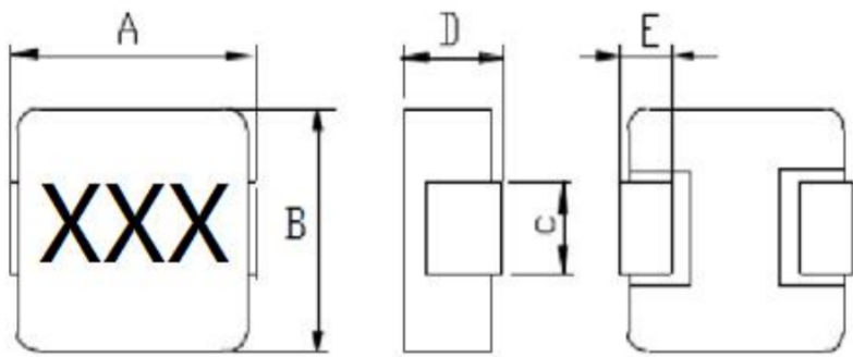
Outline Dimensions 外形尺寸
