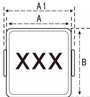
Outline Dimensions 外形尺寸
