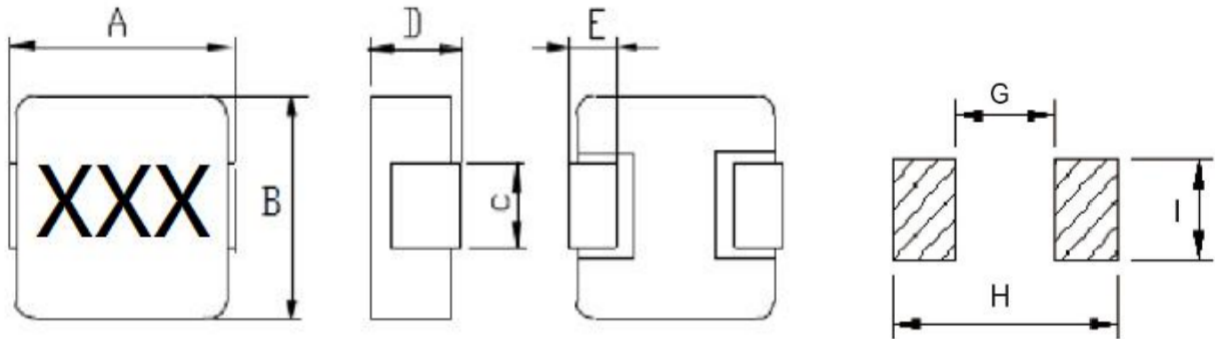
Outline Dimensions 外形尺寸
